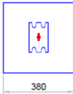
Lyftögla M16
